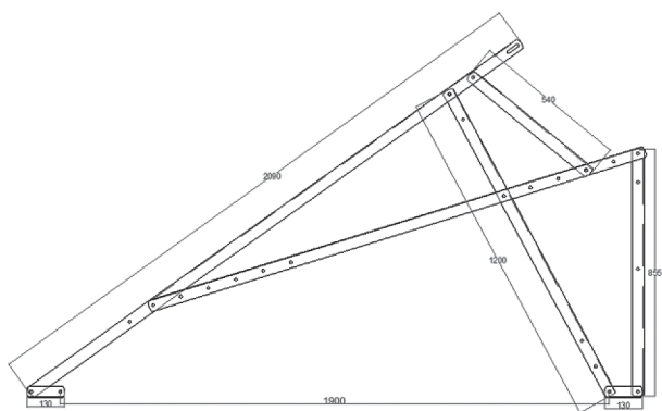
PERFIL IZQUIERDO
