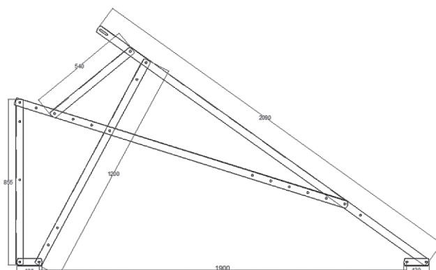
PERFIL DERECHO
